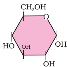
C_6H_{12}O_6 (ग्लूकोज)
